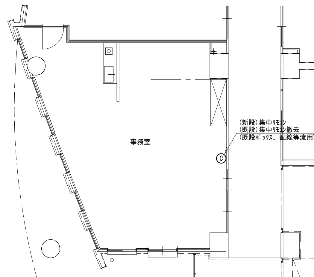
② 西棟 1階平面図 S=1/100
